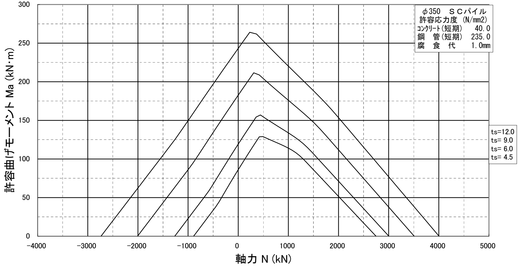
許容曲げモーメント-軸力相関図 SCパイプ φ350
