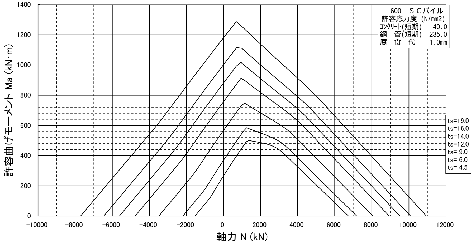
許容曲げモーメント-軸力相関図 SCパイプ φ600
