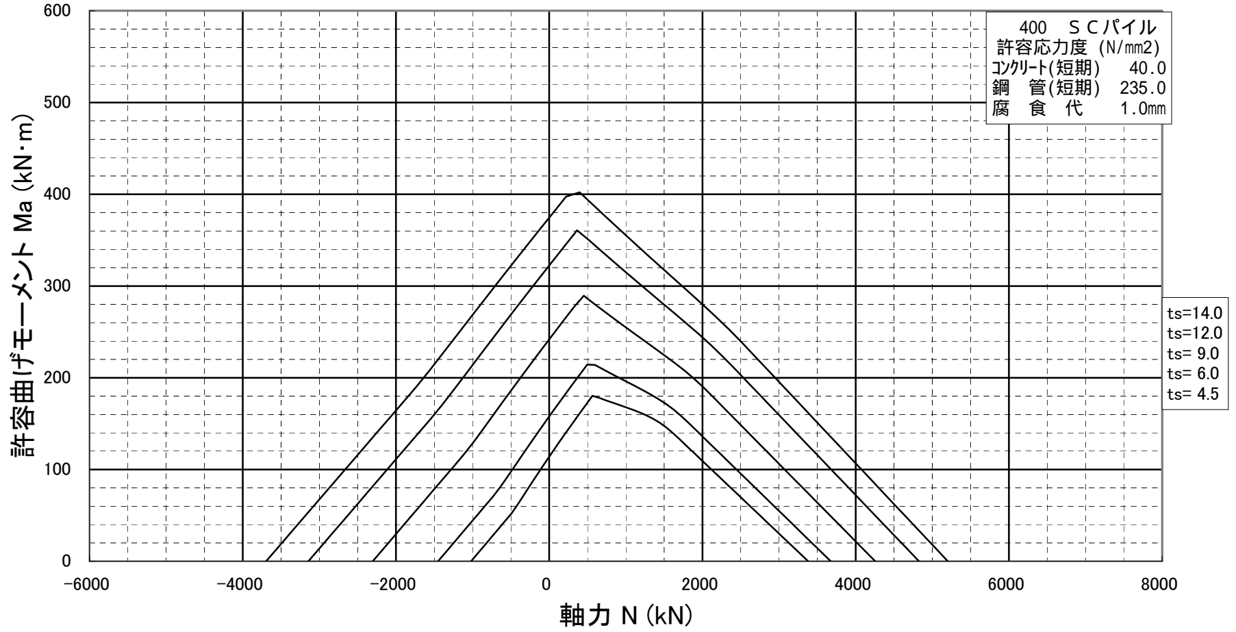
許容曲げモーメント-軸力相関図 SCパイプ φ400
