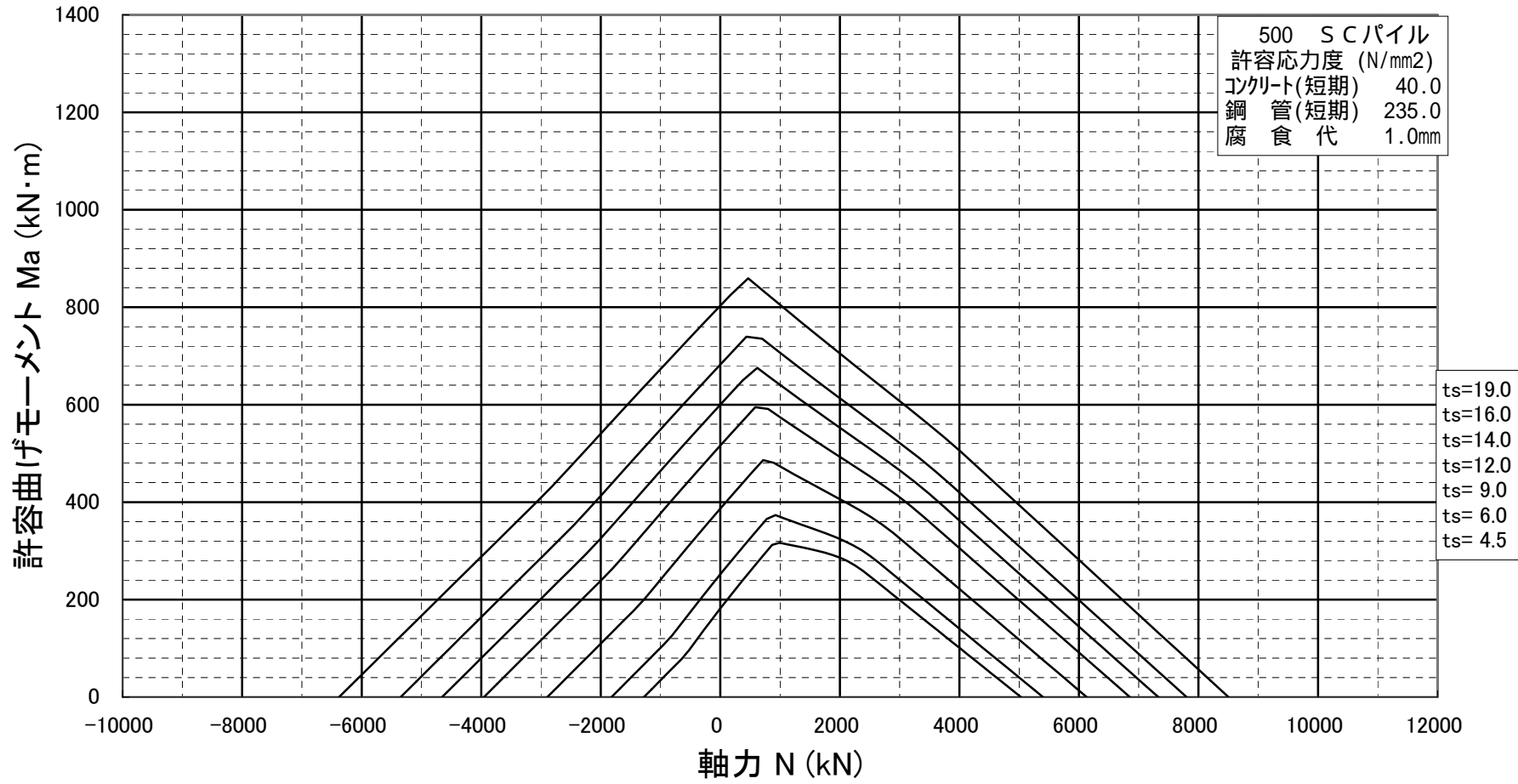
許容曲げモーメント-軸力相関図 SCパイプ φ500
