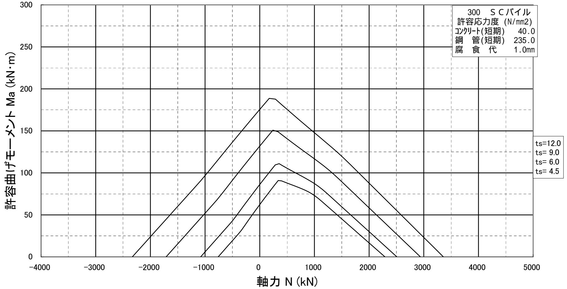
許容曲げモーメント-軸力相関図 SCパイプ φ300
