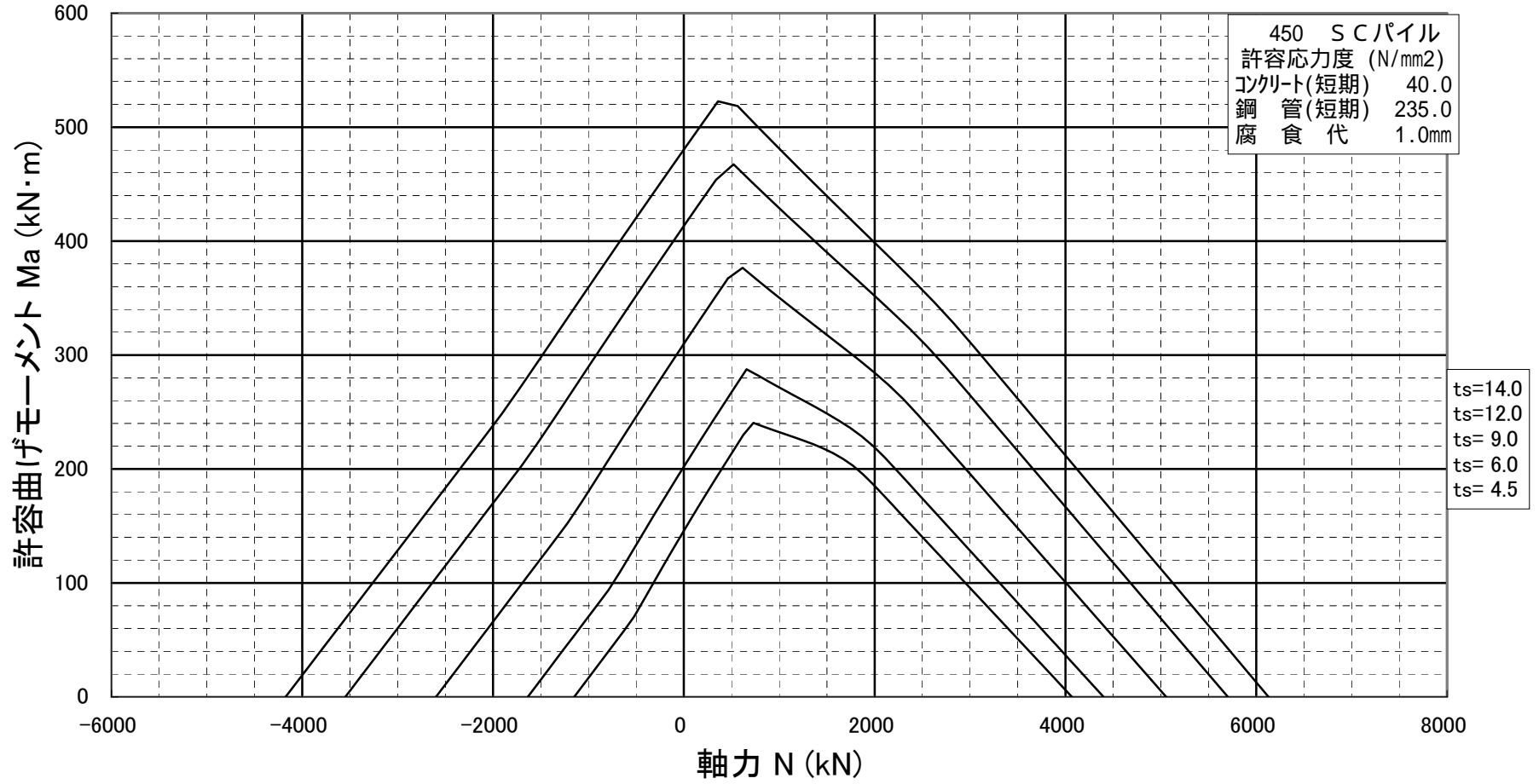
許容曲げモーメント-軸力相関図 SCパイプ φ450
